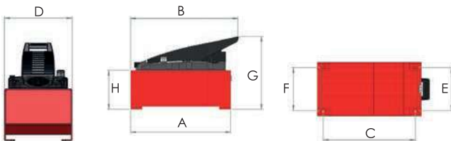
AHP1121, AHP1141 (depósito de aceite hecho de metal)
