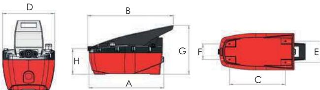
AHP1120 (depósito de aceite hecho de plástico)
