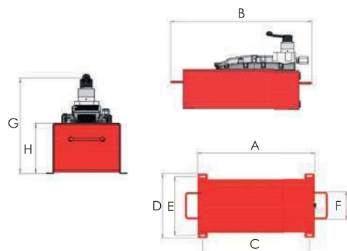
AHP1122, AHP1142 (depósito de aceite hecho de metal)
